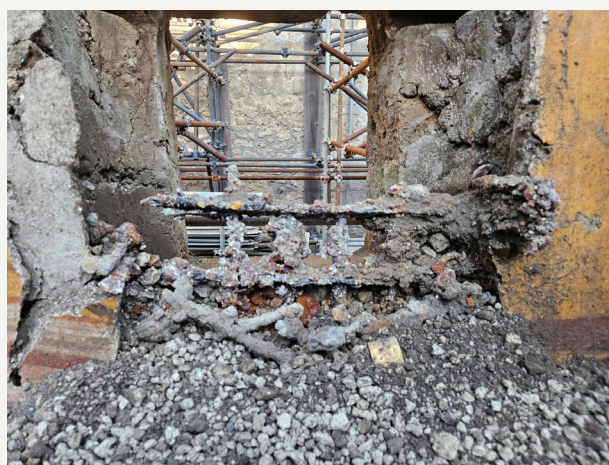
FIG. 31 Ambiente B1, parete est. Particolare della grata in ferro della finestra che affaccia sul vicoletto di divisione delle insule. Da ovest.
